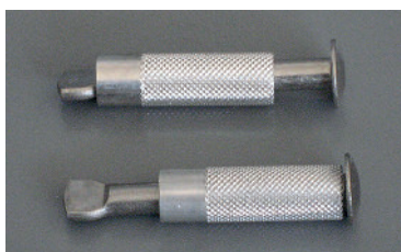
Pitons escamotables
